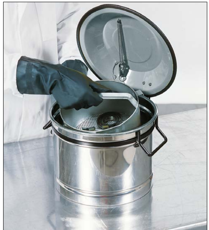
① Edelstahl-Tränkbehälter, 2,5 Liter, serienmäßig mit Flamm Sperre, Bestell-Nr. 117-256-J0
