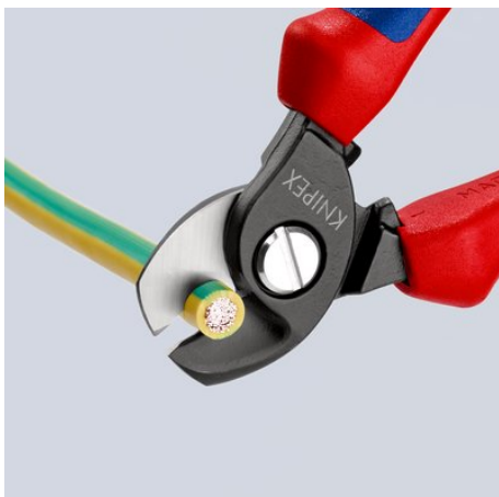
Cięcie za pomocą nożyce do kabli: łatwe, czyste cięcie bez deformacji kabla
