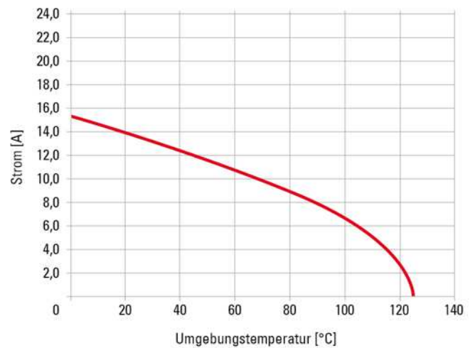
Stromtragfähigkeit Schirm max. 14A at 20°C 80 polig, Bauform low
