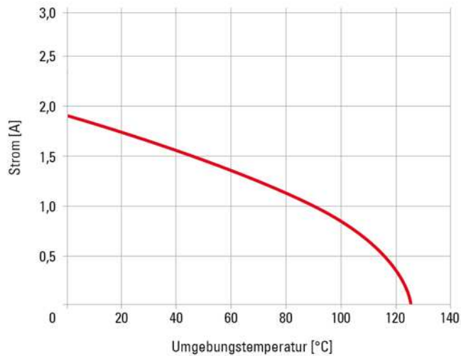
Stromtragfähigkeit Signalkontakte max. 1.7A bei 20°C (80 polig)
