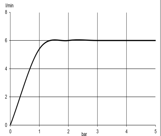
Durchflussdiagramm
