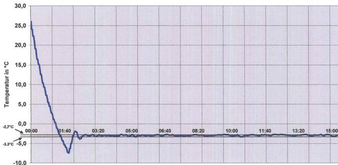
Regelverhalten Beispiel: Zieltemperatur -3^{\circ}\text{C}
