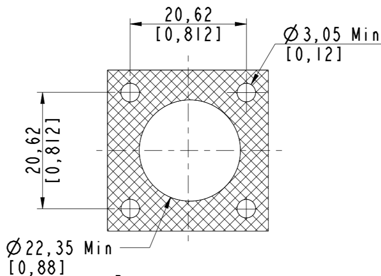
Perçage panneau Panel drilling
