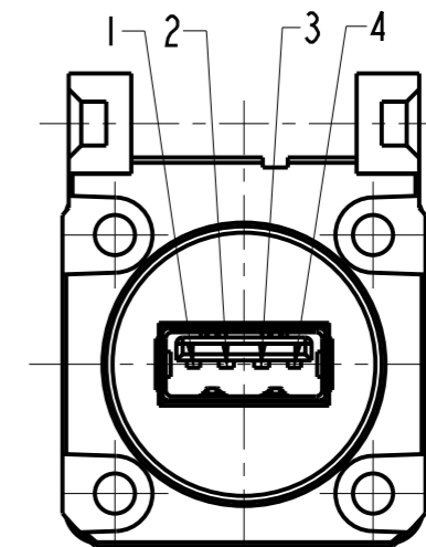
USB-A Vue B avant sans bouchon Front view B without cap
