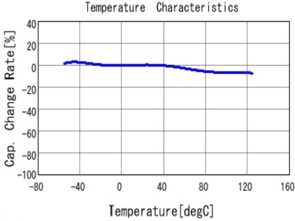
■ GCJ188R71E103KA01 C-Temp. capchange, DCO. 0V, AC1.0V rm
