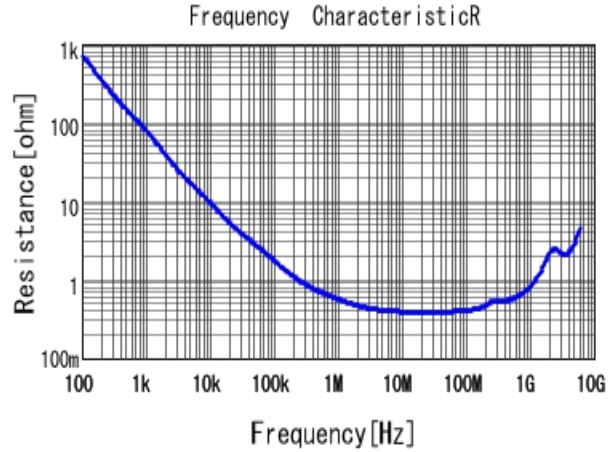
■ GCJ188R71E103KA01 R DCOV, 25degC
