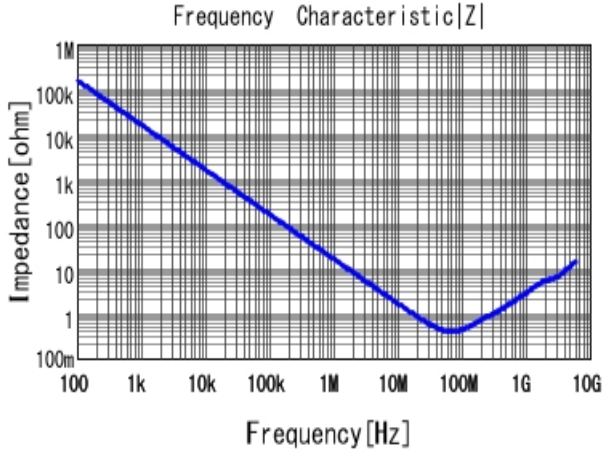
■ GCJ188R71E103KA01 |Z| DCOV, 25degC
