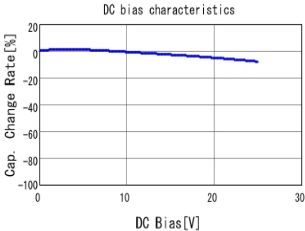
■ GCJ188R71E103KA01 C-DC bias capchange, 25.0degC, AC1.
