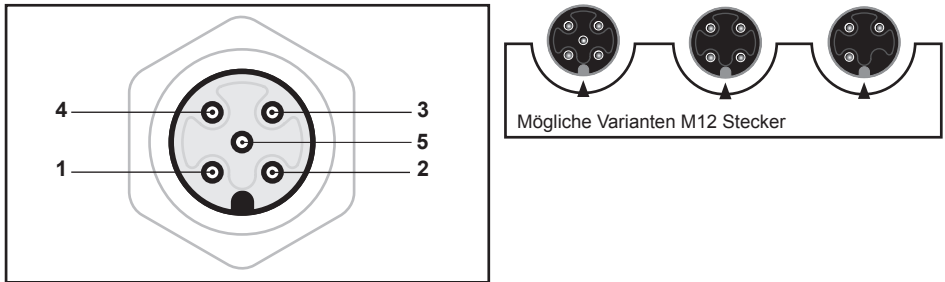
Schemazeichnung M12-Stecker
