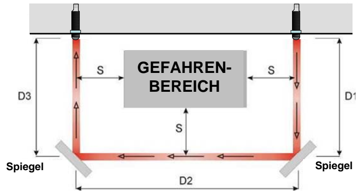
Abb. 11 Umlenkspiegel
