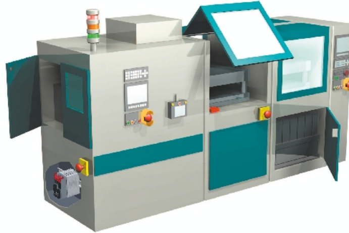
Abb. 4 Kontrolle von Öffnungen über Sicherheitsfotозellen
