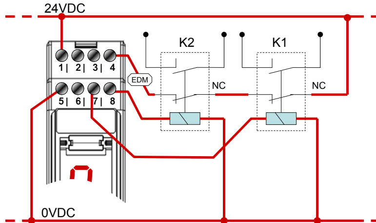
Abb. 16 EDM-Anschlusschema
