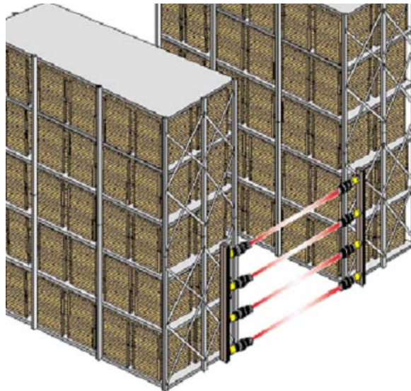
Abb. 3 Schutz der Zugänge in Gefahrenbereiche durch Sicherheitsfotозellen
