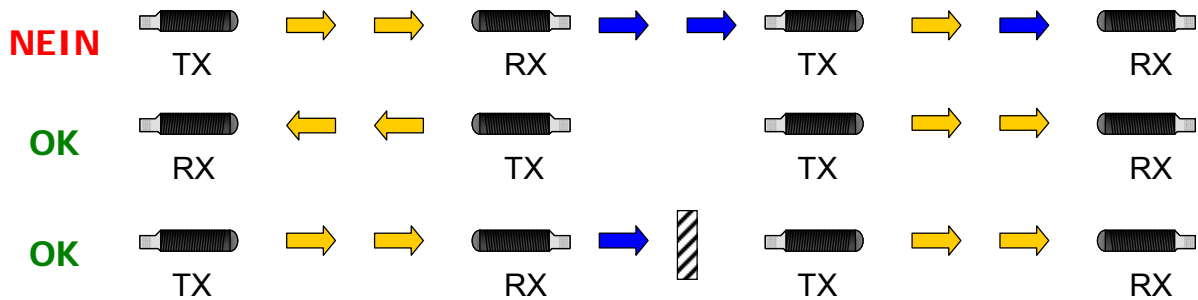
Abb. 8 Anordnung der Sensoren zur Vermeidung von Interferenzen
