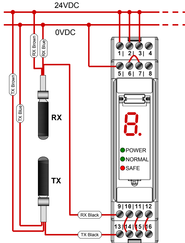
Abb. 13 Mindestanforderung an den Anschluss zur Funktionskontrolle
