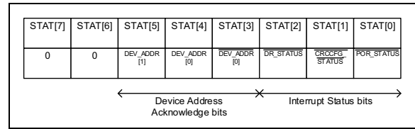
FIGURE 6-1: STATUS Byte.
