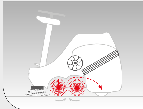
Die gegenläufigen Kehrwalzen des Doppel-Walzen-Systems befördern Kehrgut in den Behälter.
