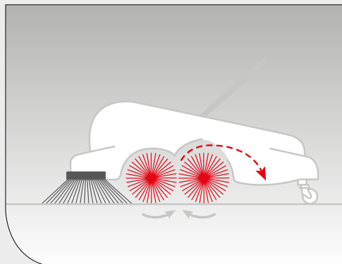
Durch das Doppel-Walzen-System wird das Kehrgut mit Hilfe der gegenläufig rotierenden Kehrwalzen aufgenommen und in den Behälter befördert.
