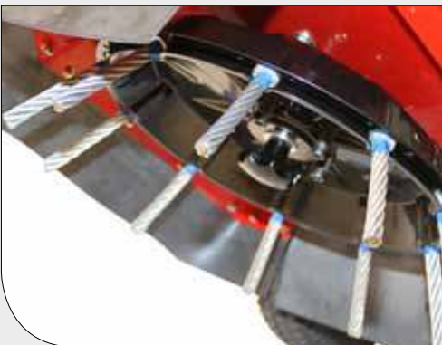
Werkzeugteller mit Schnellwechselsystem zum Borsenwechsel.
