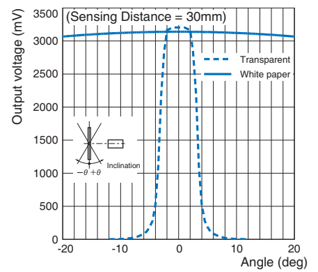
B5W-LB2101
