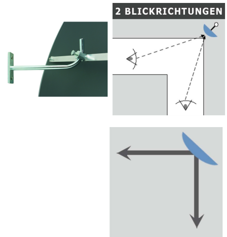
Modellbeispiel: Beobachtungsspiegel -Detektiv-A-, aus schlagfestem Acrylglas (Art. 11260)
