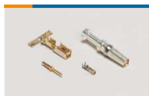
Steckverbinderkontakte(12)
