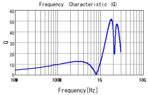
■ LQG15HHR12J02 Q
