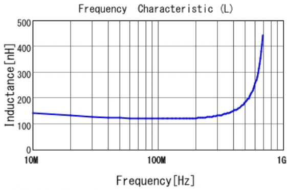
■ LQG15HHR12J02 L
