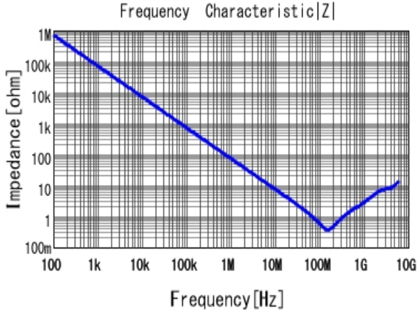
■ GCJ188R71E222KA01 |Z| DCOV, 25degC
