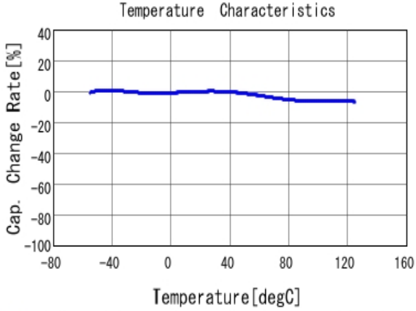
■ GCJ188R71E222KA01 C-Temp. capchange, DCO. 0V, AC1.0V r m
