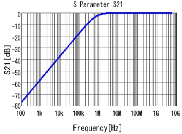
■ GCJ188R71E222KA01 S21 DCOV, 25degC
