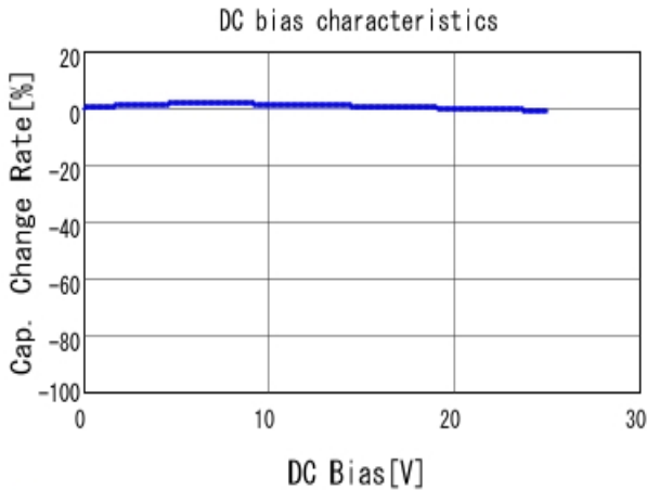
■ GCJ188R71E222KA01 C-DC bias capchange, 25.0degC, AC1.
