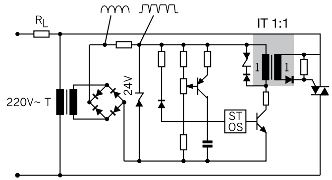
Triac-Phasenanschnittsteuerung
