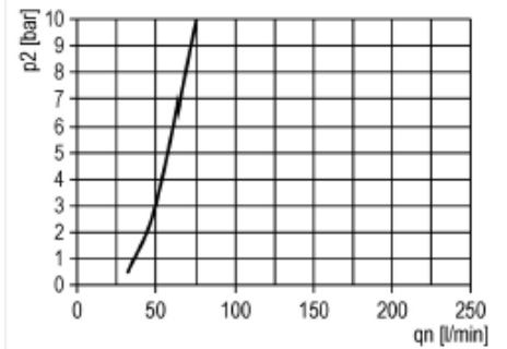
Öleransprechgrenze
