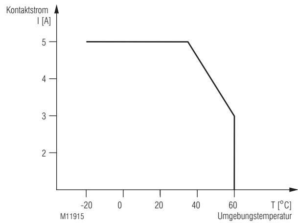
Dauerstrom-Grenzkurve IK 3070.12
