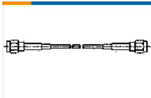
TE Teilenummer1337808-1 50 OHM COAX SMA STR PLUG STR P
