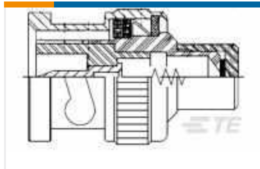
TE Teilenummer1-1337463-0 BNC Plg Term 50Ohm Silver Pltd
