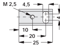
SK 12 SA 32 30 K/W 1 x SOT 32
