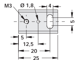
UK 14 SA M3
