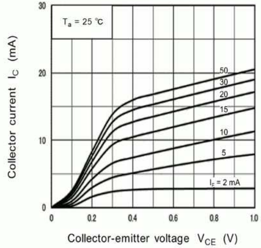
Fig. 11.8 I_C - V_{CE0}
