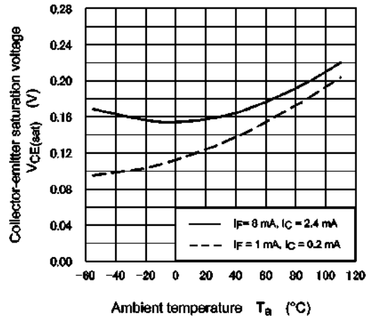
Fig. 11.10 V_{CE(sat)} - T_a
