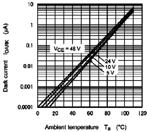
Fig. 11.9 I_{DARK} - T_a
