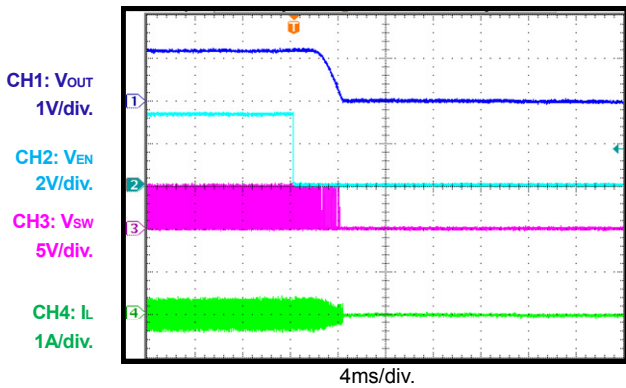
EN Off I_{OUT} = 0A
