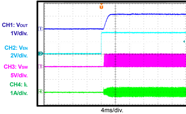
EN On I_{OUT} = 0A
