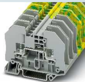
24 A, Durchgangsklemme, offen
