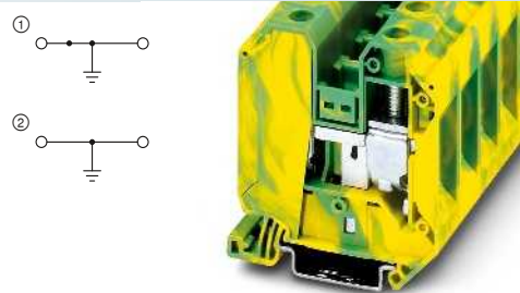
125 A, Schutzleiterklemme
