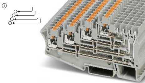
10 A, Vierstockklemme
