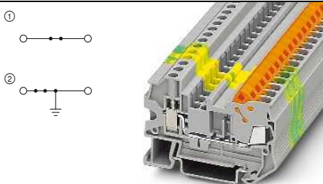
24 A, Durchgangsklemme
