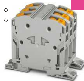
150 A, Klemmenblock zur Direktmontage
