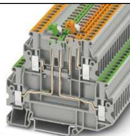
16 A, Doppelstockklemme mit Trennmesser je Etage, Prüfbuchenschraube
