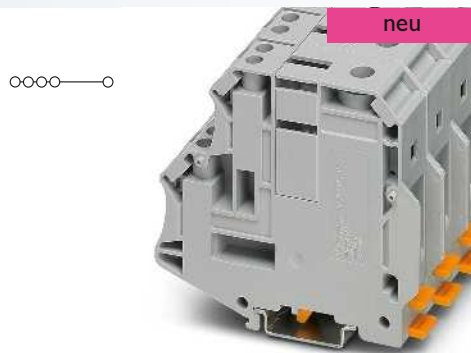
192 A, Einspeiseklemme, 4 Abgänge 10 mm 2
