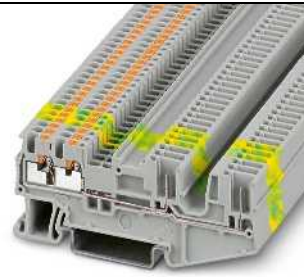
17,5 A, Durchgangsklemme, 4 Anschlüsse
