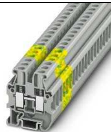
41 A, Durchgangs- und Schutzleiterklemme
