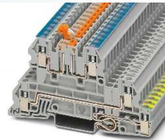
4 (4) mm 2 , 24 A, Dreistockklemme, 1 x Außenleiter L, 1 x N-Leiter trennbar, 1 x PE
