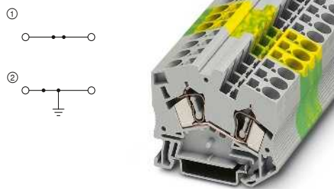
57 A, Durchgangsklemme
