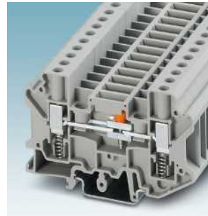
Federunterstützte Trennklemmen USST-T ...
