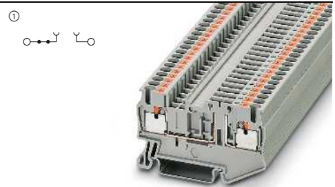
20 A, Trennklemme, mit 2 Funktionsschächten
