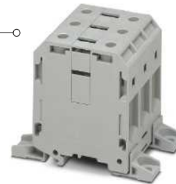
192 A, Klemmenblöcke zur Direktmontage
