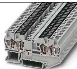
17,5 A, Durchgangsklemme, 4 Anschlüsse, mit unterbrochenem Strombalken
