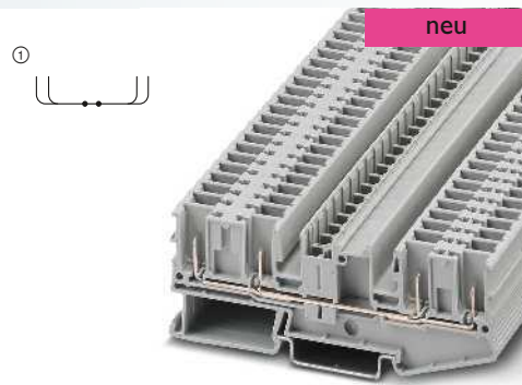
32 A, Durchgangsklemme, 4 Anschlüsse
