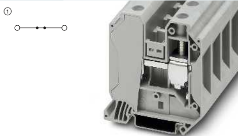
150 A, Durchgangsklemme
