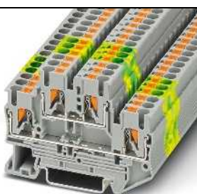
26 A, Doppelstockklemme, 4 Anschlusse
