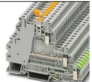
36 A, Mehrstockklemme mit Messertrennzone, PE-Fuß
