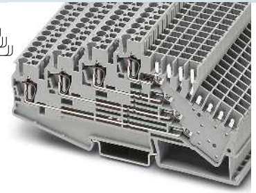
10 A, Vierstockklemme, zwei Steckplätze
