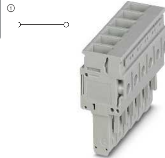
41 A, Stecker, Anschluss in Steckrichtung
