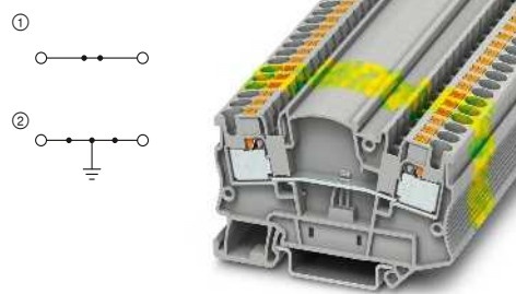
32 A, Durchgangsklemme, konturgleich
