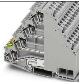
32 A, Vierstockklemme mit PE-Fuß
