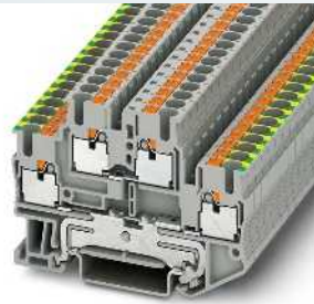
30 A, Doppelstockklemme mit PE-Fuß
