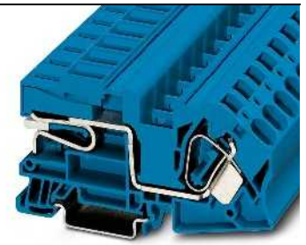
76 A, N-Trennklemme
