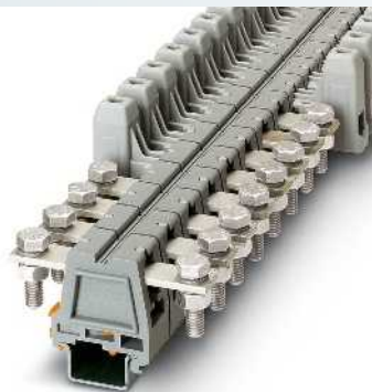
25 (25) mm 2 , 101 A, Durchgangsklemme
