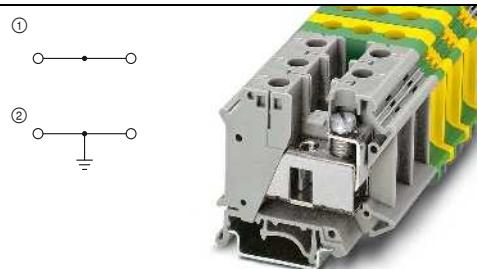
125 A, Durchgangs- und Schutzleiterklemme
