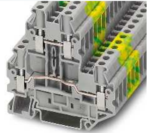
36 A, Doppelstock- und Schutzleiterklemme
