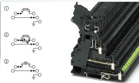
36 A, Mehrstockklemme, Sicherungshebel mit Leuchtanzeige, PE-Fuß
