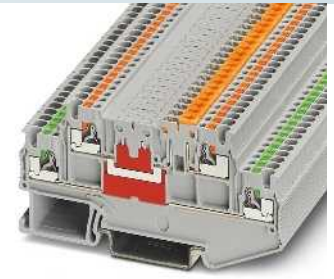
9 A, Messertrenn-Doppelstockklemme, obere Etage trennbar
