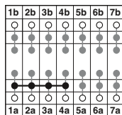
Prüfstecker Typ B7
