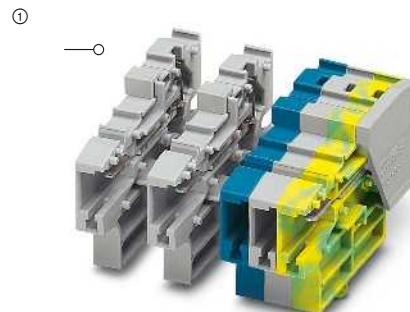
32 A, Kupplung mit Rastzapfen, selbstkonfigurierbar
