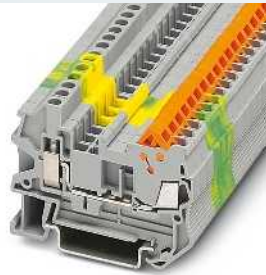
17,5 A, Durchgangsklemme
