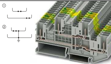
22 A, Doppelstockklemme
