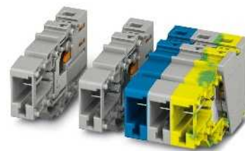
41 A, Kupplung, selbstkonfektionierbar
