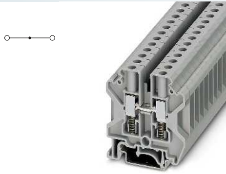
6 (10) mm 2 , 57 A, Durchgangsklemme
