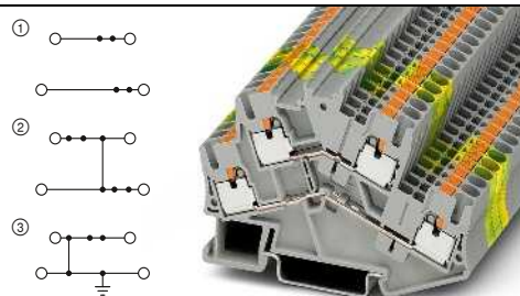
24 A, Doppelstockklemme
