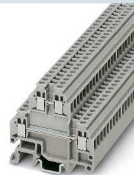
1,5 (1,5) mm 2 , 17,5 A, Doppelstockklemme
