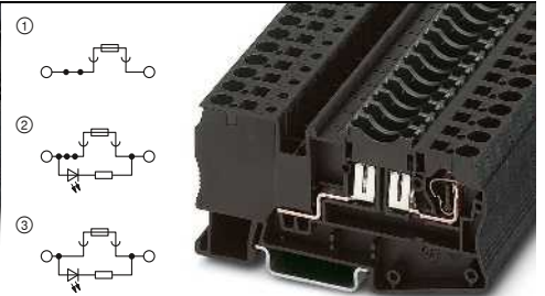
30 A, Sicherungsklemme für Flachsicherungen Typ C
