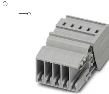
24 A, Kupplung
