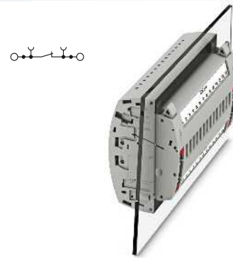
6 (10) mm 2 , 30 A, Prüfsteckleiste, VDE kodiert Typ A14
