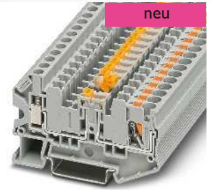
20 A, Messertrennklemme, 3 Funktionsschächte und zwei 4-mm-Prüfbuchsen
