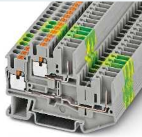
22 A, Doppelstockklemme
