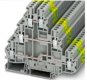
24 A, Dreistock- und Schutzleiterklemme
