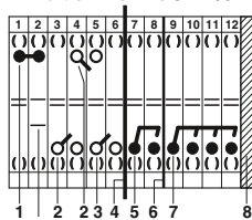
Prüftrennklemme URTK/S
