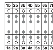
Prüfstecker Typ E7
