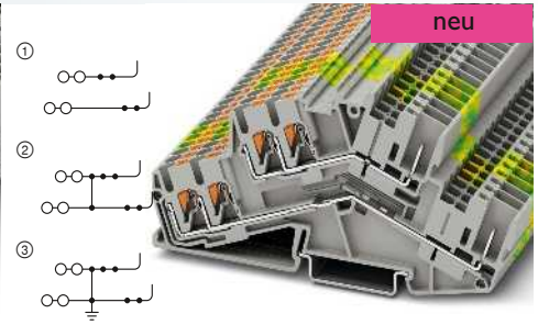
22 A, Doppelstockklemme, Pultbauform
