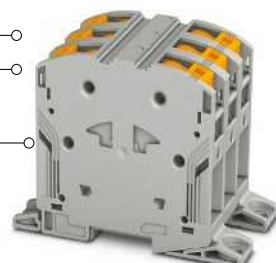
232 A, Klemmenblock zur Direktmontage
