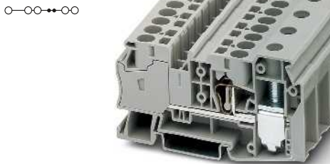
125 A (Schraubanschluss), Einspeiseklemme, 4 Abgänge 10 mm 2
