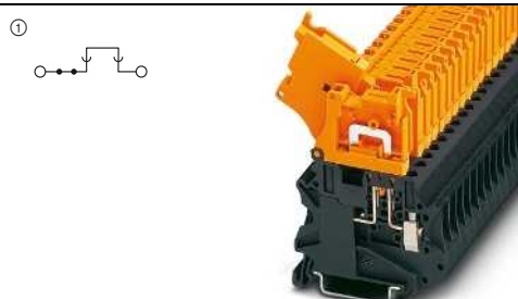
20 A, Hebeltrennklemme, konturgleich
