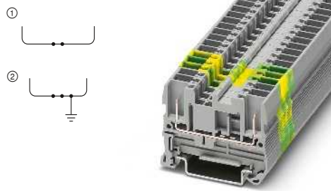
24 A, Durchgangsklemme
