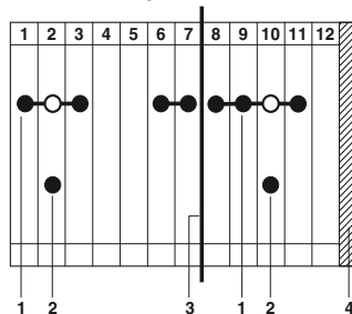
Gleitstegklemme UGSK/S
