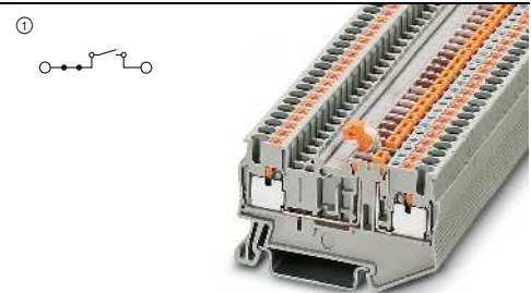
20 A, Messertrennklemme, 2 Funktionsschächte
