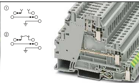
36 A, Mehrstockklemme mit Trennzone, PE-Fuß
