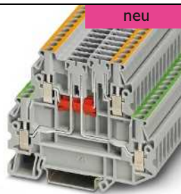
16 A, Doppelstockklammer mit zwei Trennzonen
