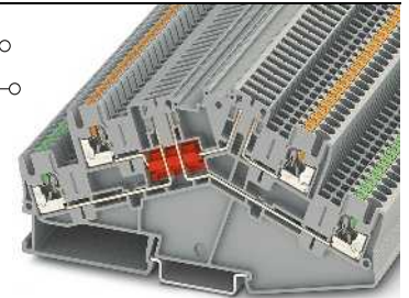
16 A, Doppelstockklemme, zwei Trennzonen
