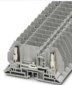
10 (10) mm 2 , 50 A, Messwandler-Trennklemme, zur Direktmontage
