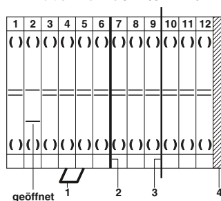
Prüftrennklemme URTK/S-BEN 10
