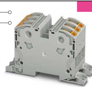
125 A, Klemmenblock zur Direktmontage
