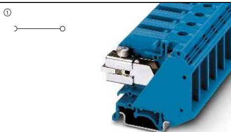
110 A, N-Trennklemme
