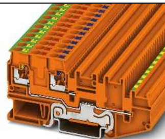
2,5 (4) mm 2 , 20 A, Einspeiseklemme mit PE-Fuß
