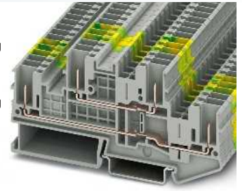
22 A, Doppelstockklemme
