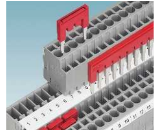
Brücken
