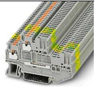
16 A, Doppelstockklemme
