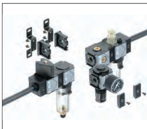
Bloccaggio "comfort". La sostituzione rapida dei componenti e delle combinazioni con il modulo di collegamento (gli anelli di tenuta sono autoadesivi) riduce i tempi di montaggio.
