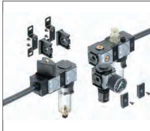
Comfortvergrendeling. De snelle ver-vanging van componenten of combinat-ies met verbindingsmodule (dicht-ringen zijn zelfklevend) verkort de mon-tagetijden.
