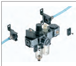
Piastre di collegamento filettate con anelli di tenuta autoadesivi (disponibili anche con angolari di tenuta) per un'installazione che supporta un facile montaggio nei sistemi di tubature sia rigide che flessibili.
