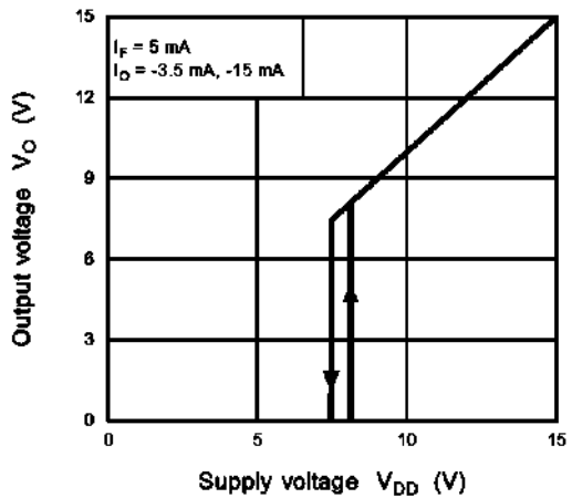
Fig. 12.2.11 V_O - V_{DD}
