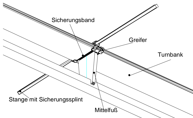
Abbildung 2: Montage
