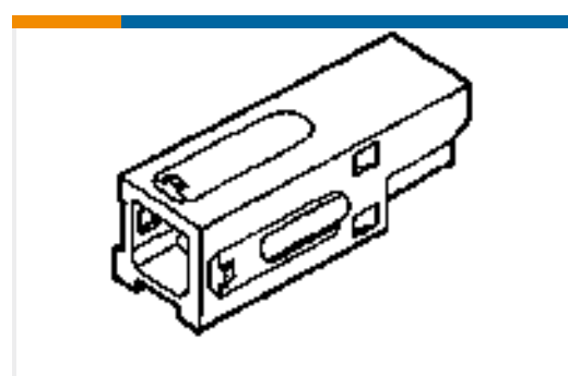
TE Teilnr.:53894-6 HSG ASSY,PWR LK,SRS1,1 POS,BLU
