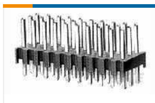
TE Teilnr.:5-103817-2 12 MODII HDR 3RST UNSHRD .100
