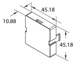
Hintere Abdeckung für 3,5 " Display
