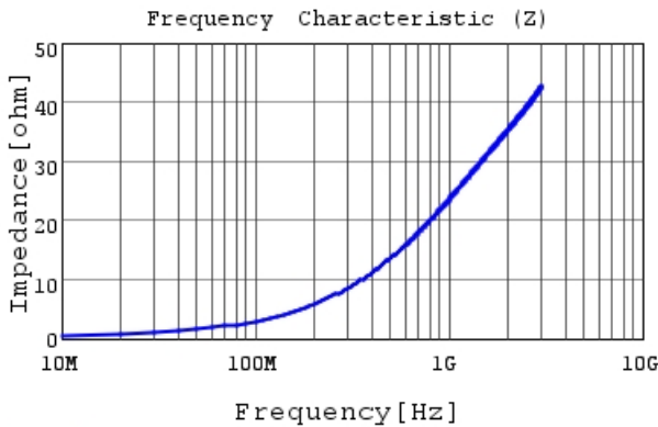
LQW18CN4N9D0H |Z|
