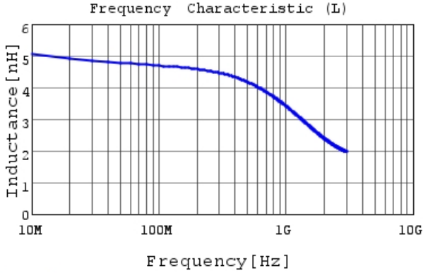
LQW18CN4N9D0H L
