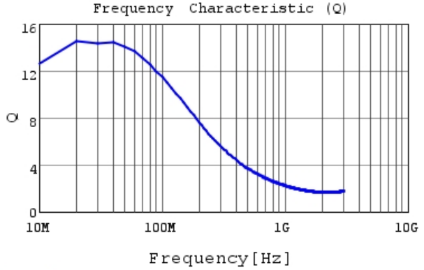
LQW18CN4N9D0H Q
