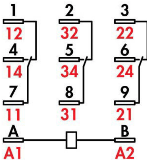
3PDT
