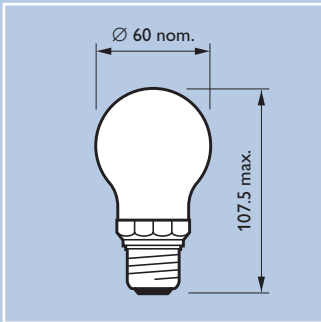
PF710E PF712E E27 Dimensions in mm
