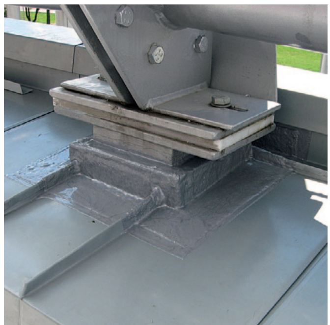
Dachaufbauten mit komplizierter Geometrie
