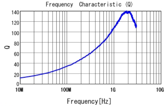
■ LQW18AN15NJ10 Q
