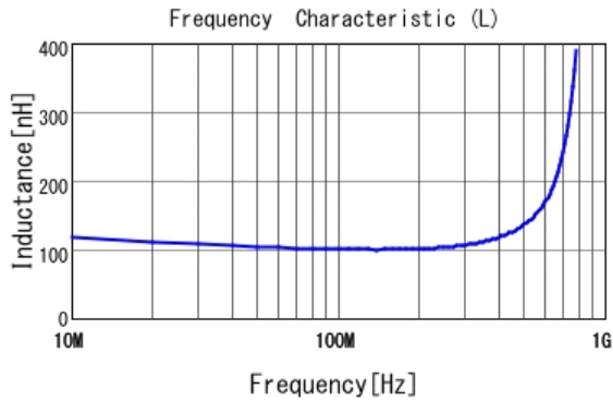
■ LQG15HZR10J02 L
