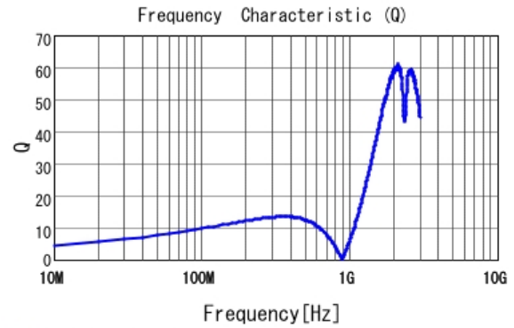
■ LQG15HZR10J02 Q
