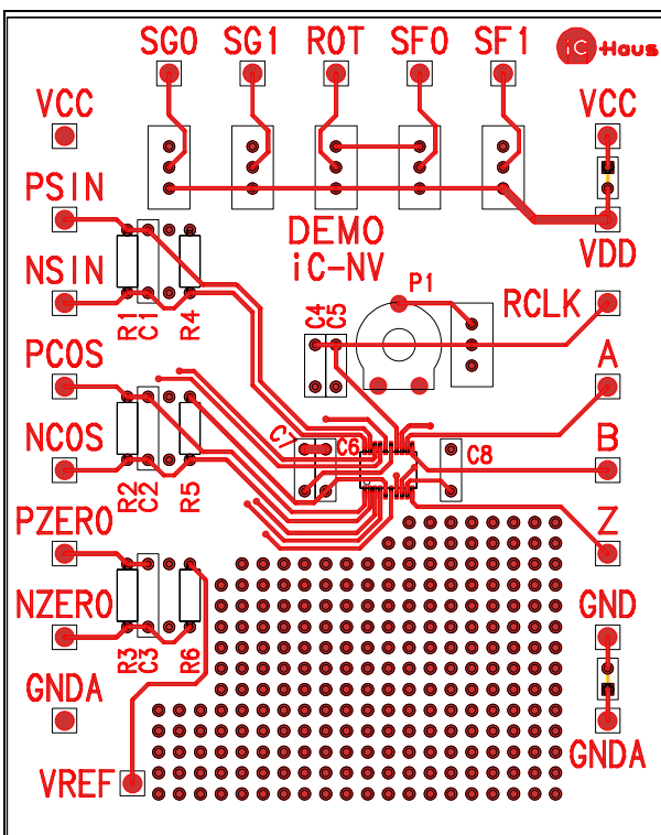
Bild 28: Demo-Board (Bestückungsseite)
