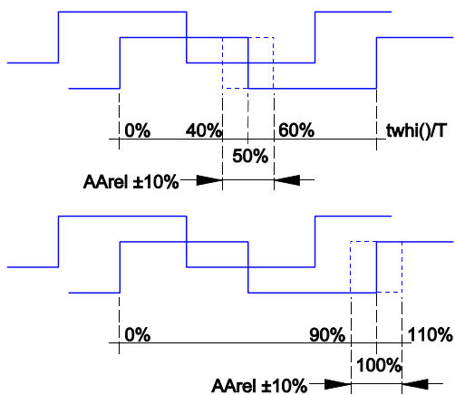
Bild 7: Definition Relativer Winkelfehler
