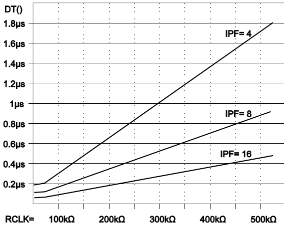
Bild 3: Einstellung des Mindest-Flankenabstands über Widerstand RCLK
