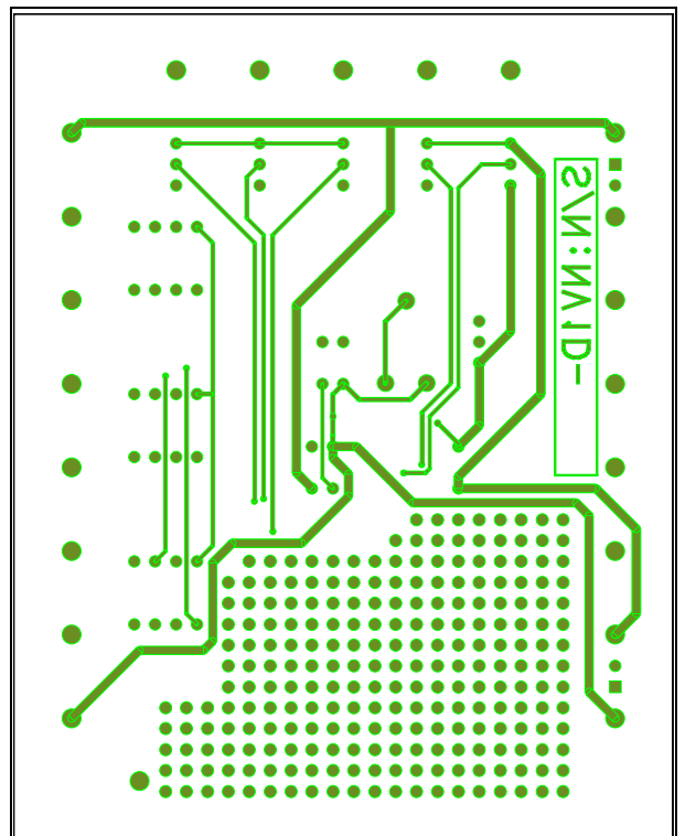
Bild 29: Demo-Board (Lötseite)
