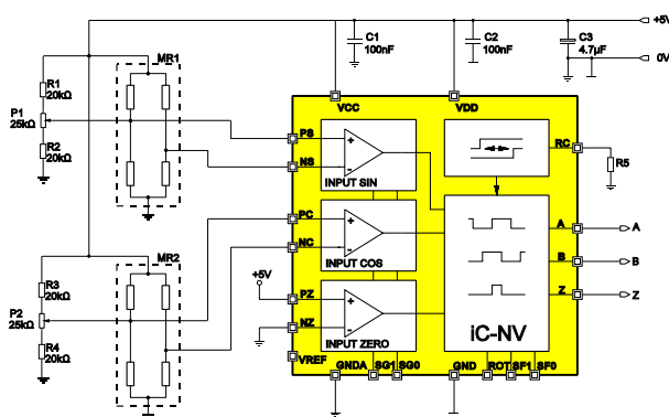
Bild 24: Anschluss von MR-Sensorbrücken mit Offset-Abgleichmöglichkeit; offene Einstellpins können zur Erhöhung der Störfestigkeit auch an VREF geschaltet werden.
