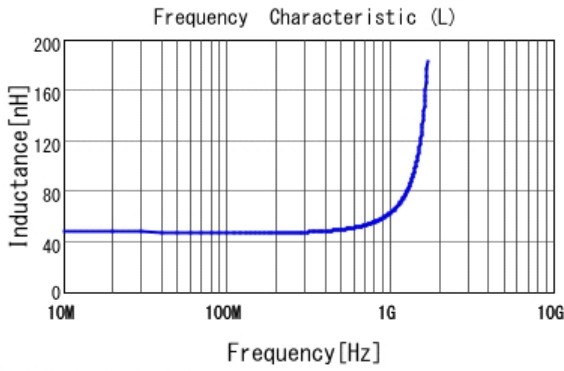
■ LQW2BAN47NJ00 L
