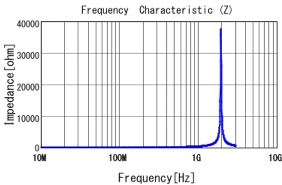
■ LQW2BAN47NJ00 |Z|
