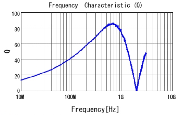
■ LQW2BAN47NJ00 Q
