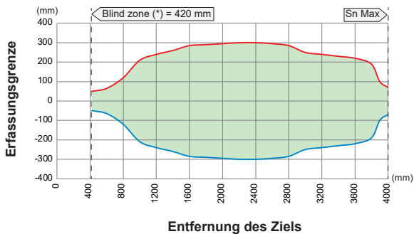
Erfassungskurve mit viereckigem Ziel 100 x 100 mm
