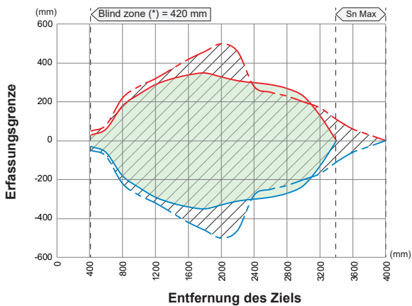
Erfassungskurve mit Rundstab
