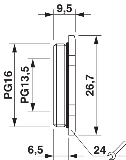
Maßzeichnung
