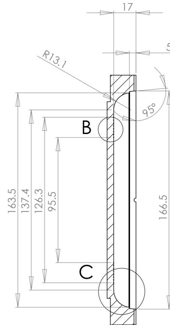
SECTION A-A
