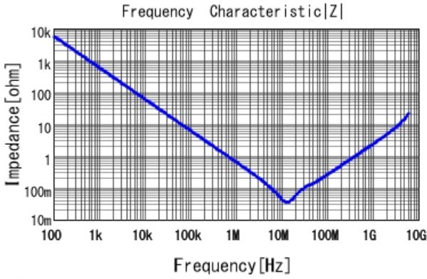
■ GCJ188R91E334KA01 |Z| DCOV, 25degC
