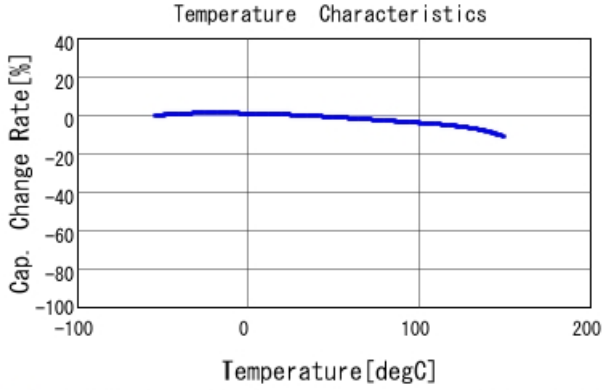
■ GCJ188R91E334KA01 C-Temp. capchange, DCO. 0V, AC1. 0Vrm
