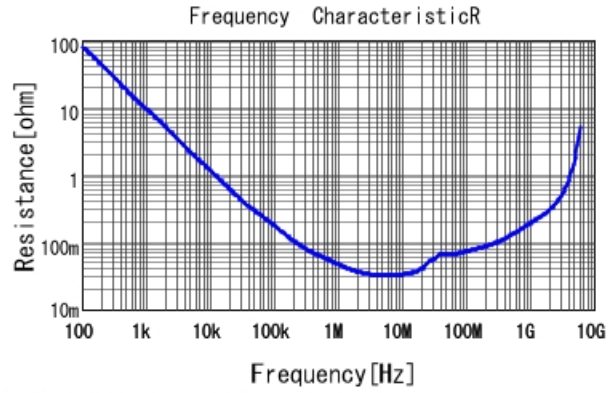
■ GCJ188R91E334KA01 R DCOV, 25degC
