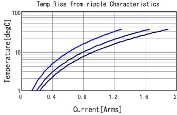
GCJ188R91E334KA01 Temp. rise ■ 300kHz ■ 600kHz ■ 1MHz
