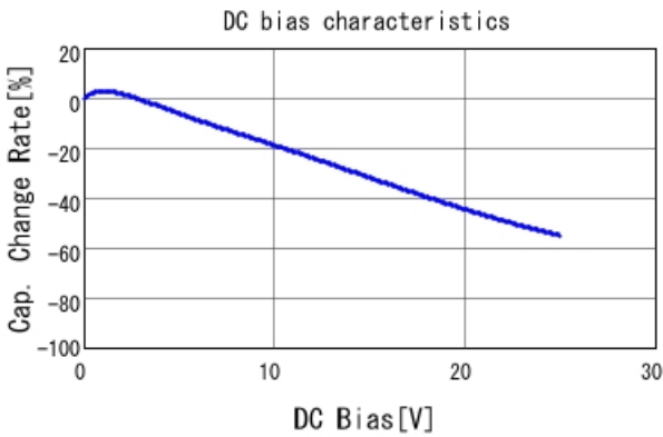
■ GCJ188R91E334KA01 C-DC bias capchange, 25.0degC, AC1.
