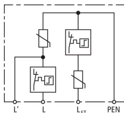
Principalschaltbild DCOR L 2P 275 SO LT
