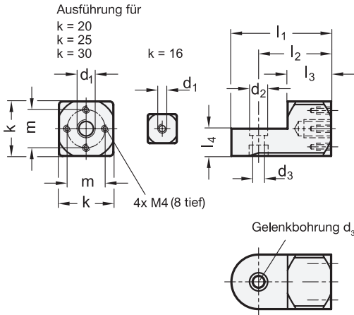
Laschengelenkset GN 511.1, Form S
