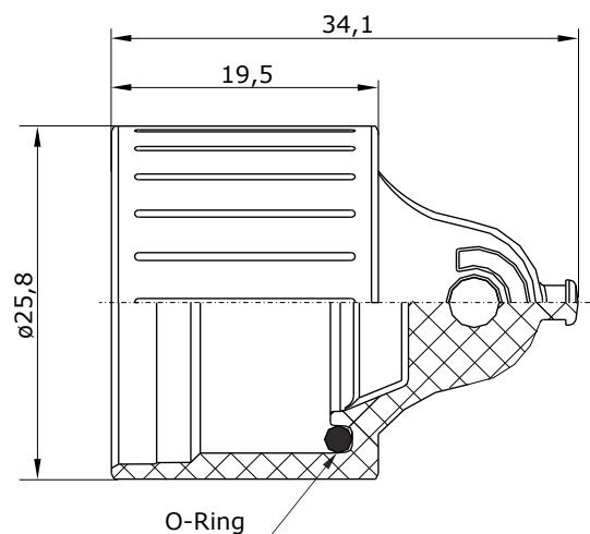
Hauptabmessungen Schutzkappe
