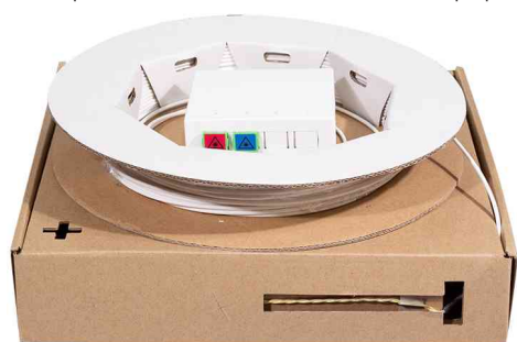
Visuel de référence : Boîte d'épissure FTTH avec câble d'installation, 2x SC / APC
