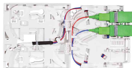
Visuel de référence : Boîte d'épissure FTTH avec câble d'installation, 2x SC / APC
