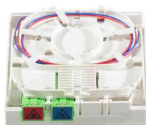
Visuel de référence : Boîte d'épissure FTTH avec câble d'installation, 2x SC / APC
