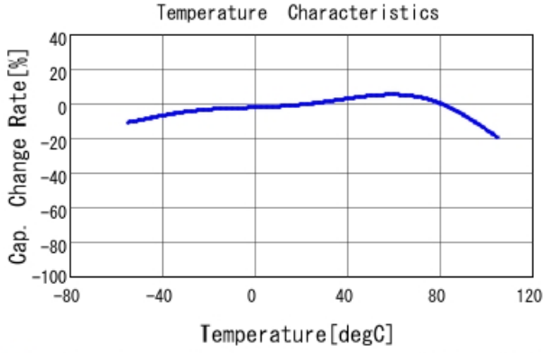
■ GRT32EC81A476KE13 C-Temp. capchange, DCO. 0V, ACO. 5Vrm
