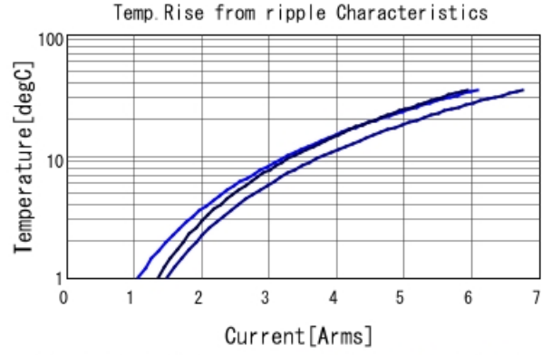
GRT32EC81A476KE13 Temp. rise ■ 60kHz ■ 300kHz ■ 600kHz
