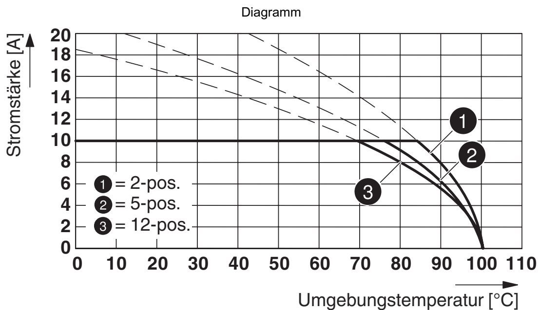
Typ: FKCN 2,5/...-ST-5,08 mit MDSTBA 2,5/...-G-5,08
