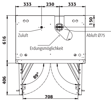
Draufsicht
