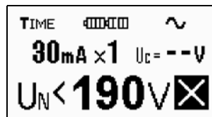
Figura 3.15 Esempio: impostazione per la misura del tempo di intervento
