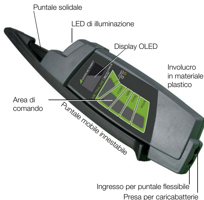
Figura 2.1 Vista dall'alto
