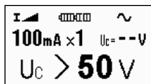
Figura 3.5 Tensione di contatto > 50\text{ V}
