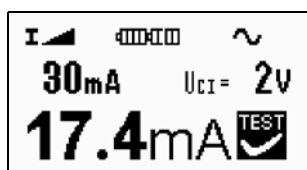
Figura 3.20 Risultato della misura della corrente di intervento
