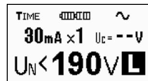
Figura 3.23 Fase applicata
