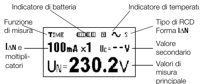
Figura 2.4 Esempio di visualizzazione
