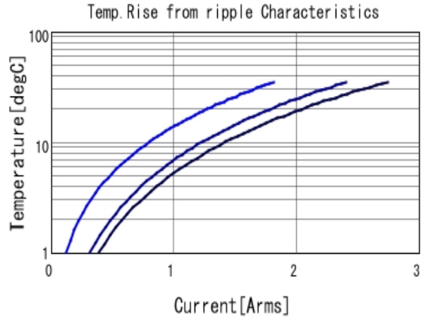
GRM033R61A105ME15 Temp. rise ■ 100kHz ■ 500kHz ■ 1MHz
