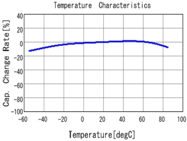
■ GRM033R61A105ME15 C-Temp. capchange, DCO. 0V, ACO. 1V rm
